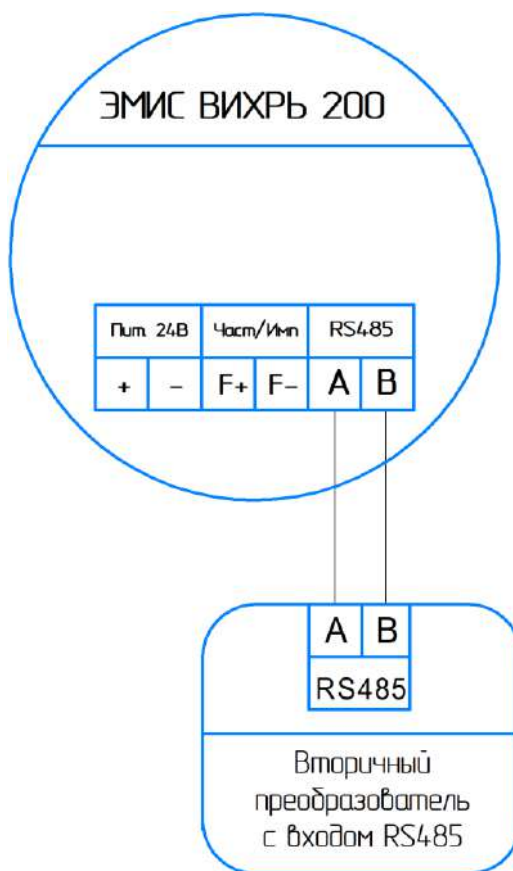
Рисунок 8.8 - Схема подключения электронного блока к вторичному оборудованию по интерфейсу RS485
