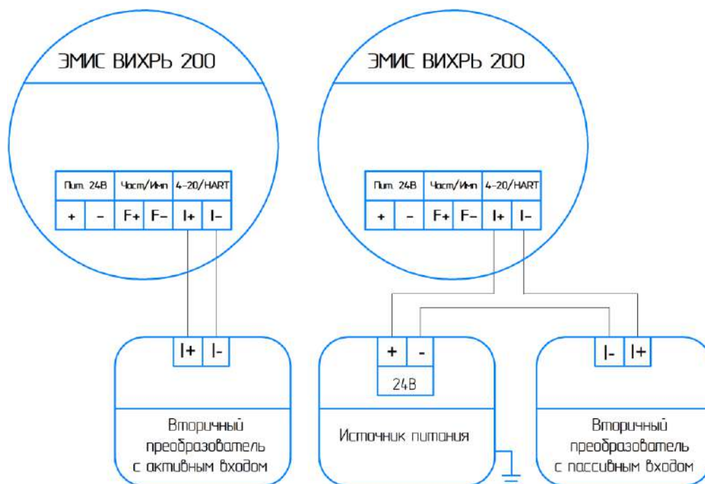
Рисунок 8.5 - Схема подключения токового выхода 4-20 мА электронного блока к вторичному преобразователю с активным (слева) и пассивным (справа) токовым входом
