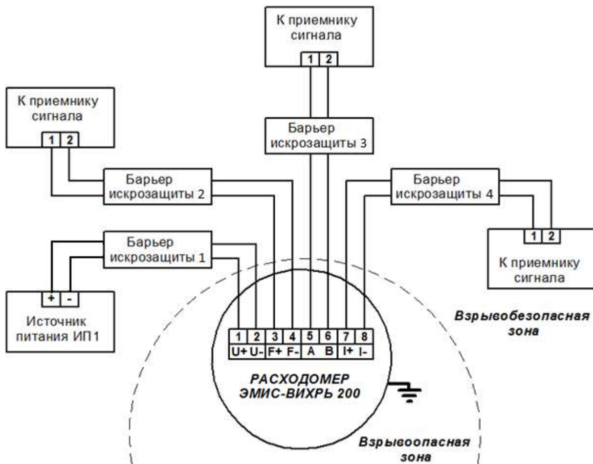
Рисунок 8.12 – Схема подключения расходомеров взрывозащищенных исполнений ExB, ExC, ExiaB, ExiaC, PVI, PO с использованием барьеров искрозащиты
