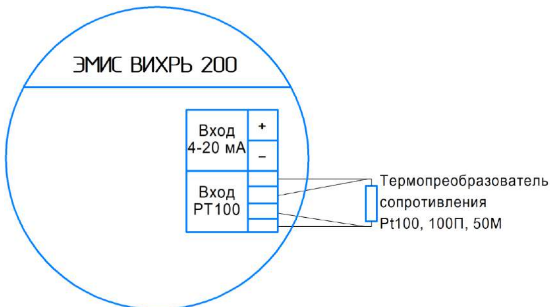
Рисунок 8.9 - Схема подключения термометра сопротивления к электронному блоку
