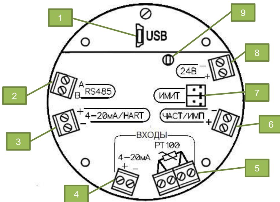
Рисунок 8.1 – Плата интерфейсов электронного блока
