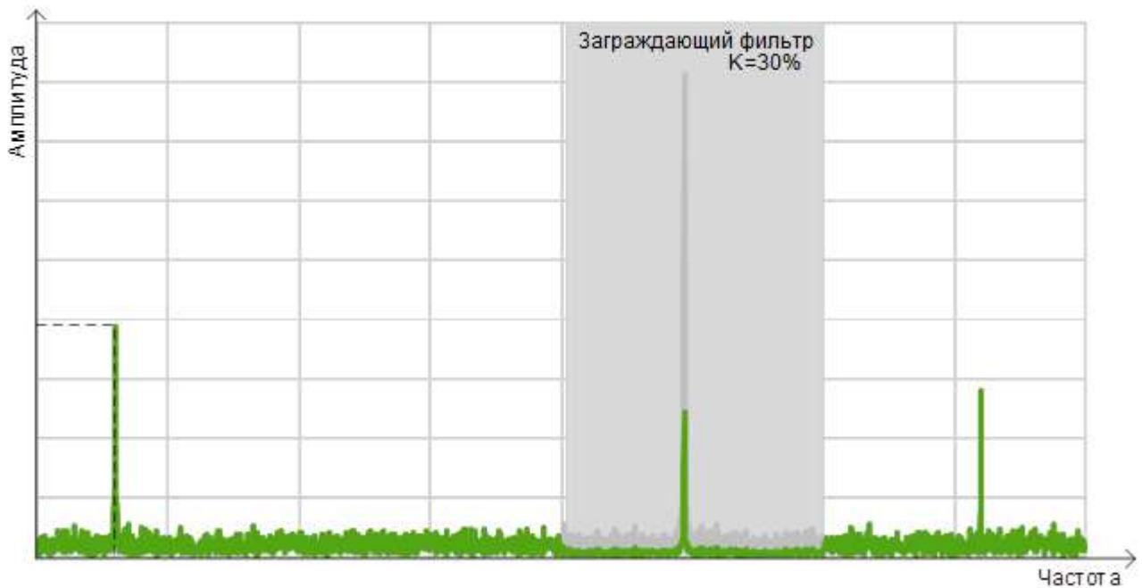
Рисунок 9.7 – Заграждающий фильтр
