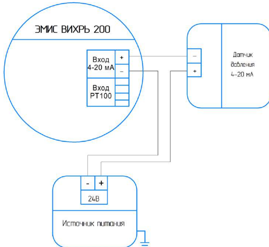
Рисунок 8.10 - Схема подключения датчика давления к электронному блоку
