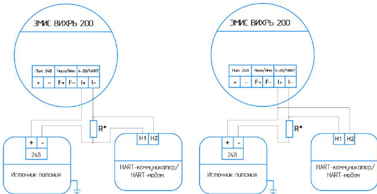
Рисунок 8.7 - Схема подключения HART-коммуникатора или HART-модема к электронному блоку для работы по протоколу HART
