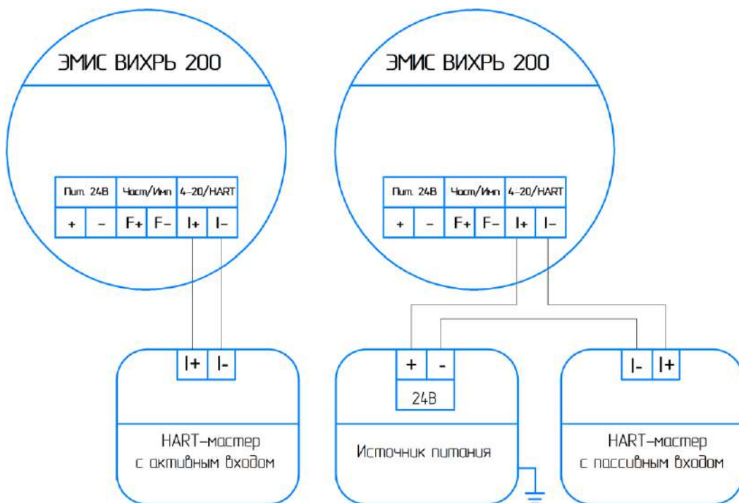
Рисунок 8.6 - Схема подключения электронного блока к HART-мастеру с активным (слева) и пассивным (справа) входом цифрового протокола HART
