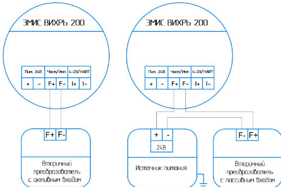
Рисунок 8.4 - Схема подключения частотно-импульсного или дискретного выхода электронного блока к вторичному преобразователю с активным (слева) и пассивным (справа) частотным входом
